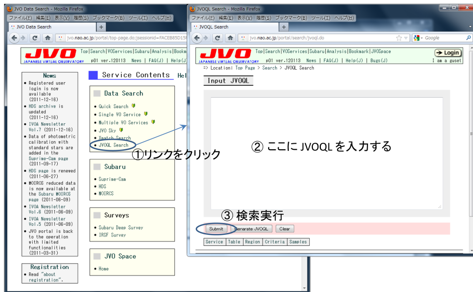
図 3: JVO portal 上での JVOQL 検索
