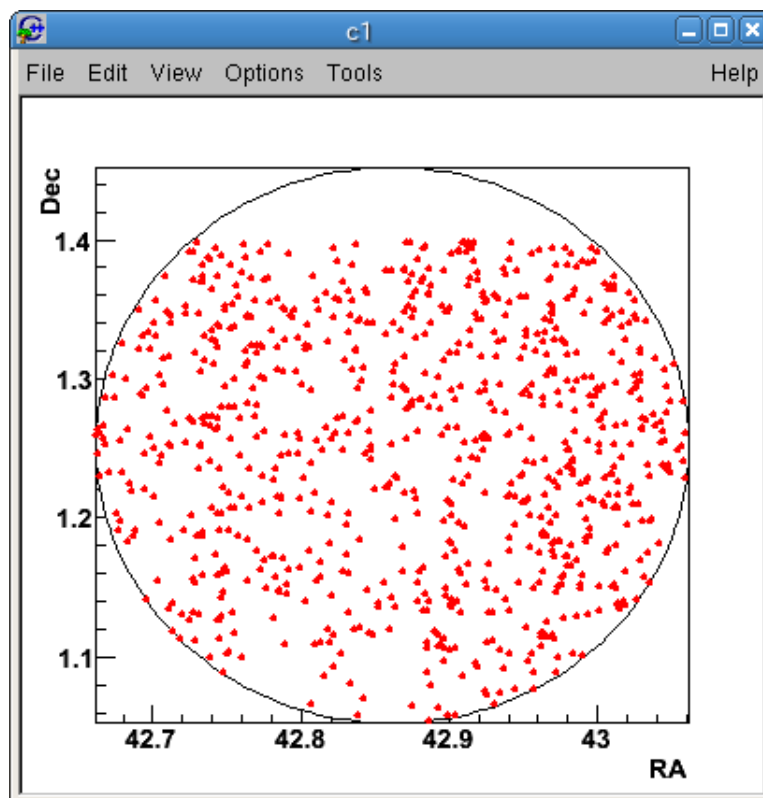
図 6: 銀河の分布。円はデータ検索範囲。
